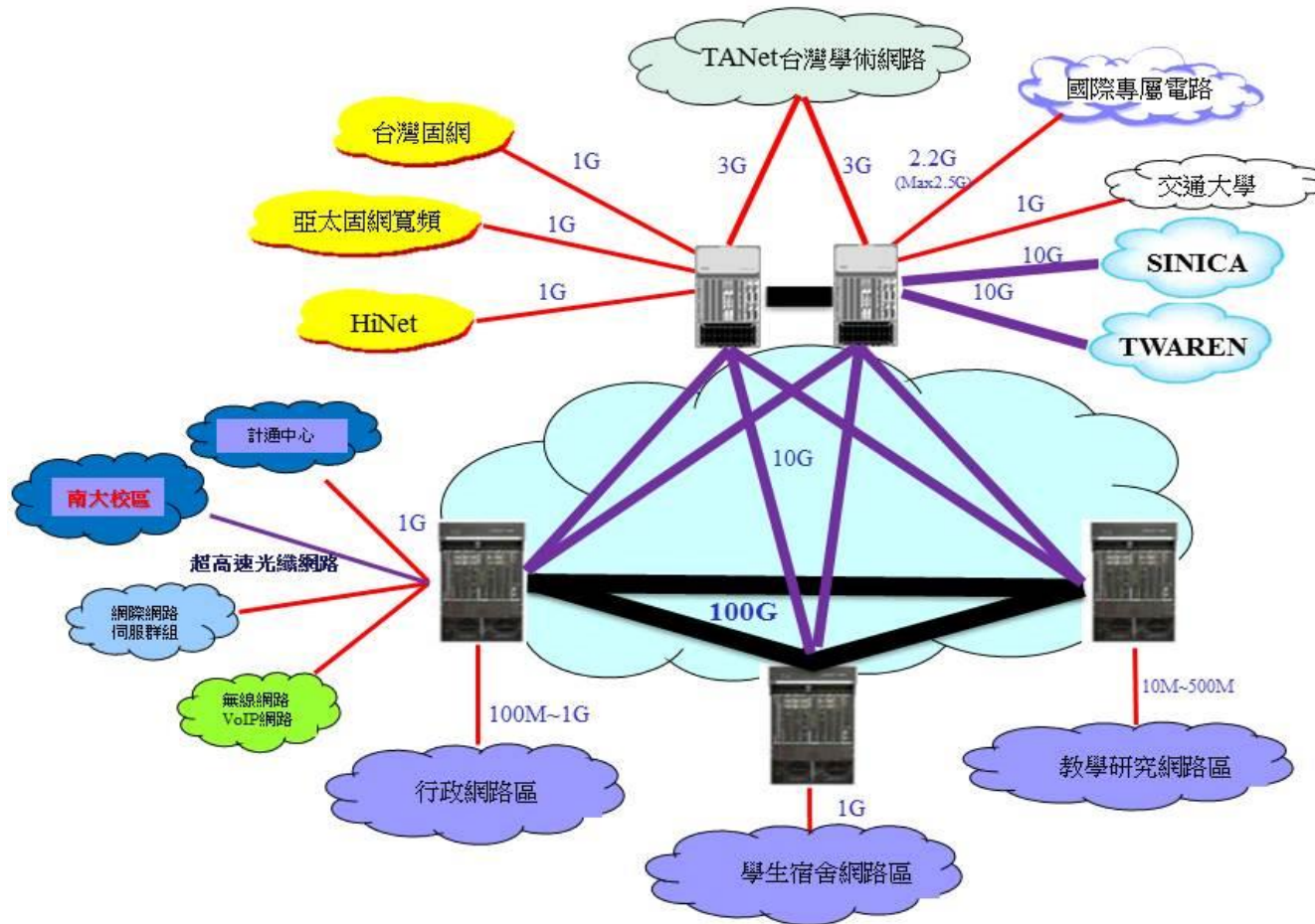
國立清華大學校園主幹網路架構示意圖
